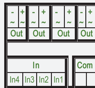
SSR-P03□-4P
