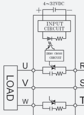
TSR-50DA-□ / TSR-75DA-□
