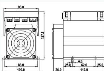
LSR-40/60/80/100 + Fan
