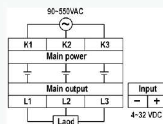
LSR-□□DA
