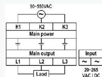
LSR-□□AA
