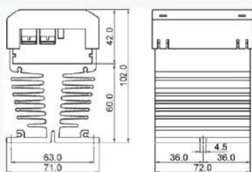
ASR-F-40/ACR-F-40
