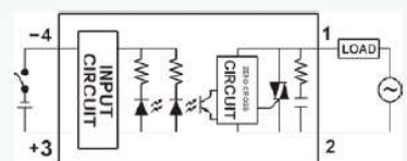
ASR-□□
