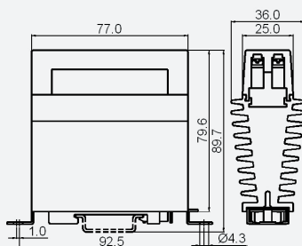
40A
