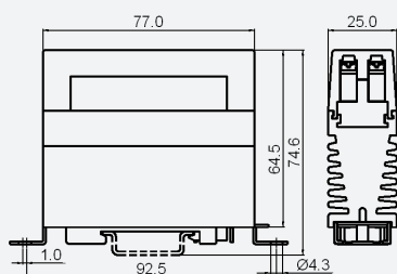
10A/20A/30A
