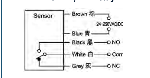
EPLS - F1 / FX Relay
