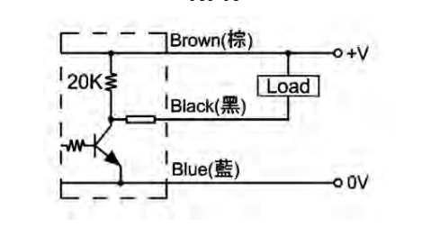
NPN
