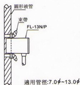
Fixed method / 安裝固定方式
